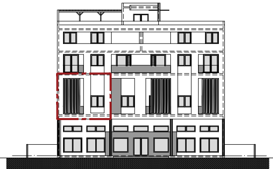
ELEVATION 1
